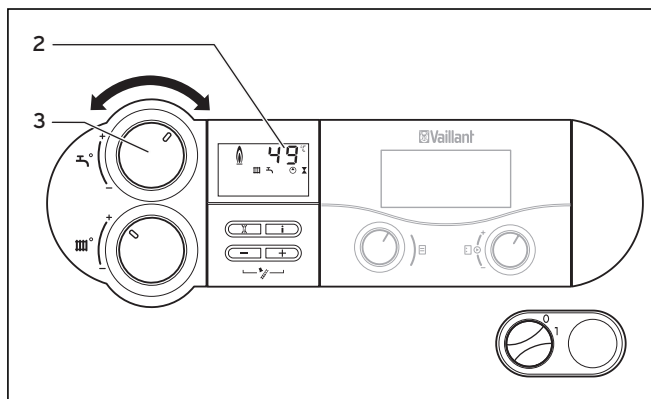
Мал. 4.6 Налаштування температури гарячої води
