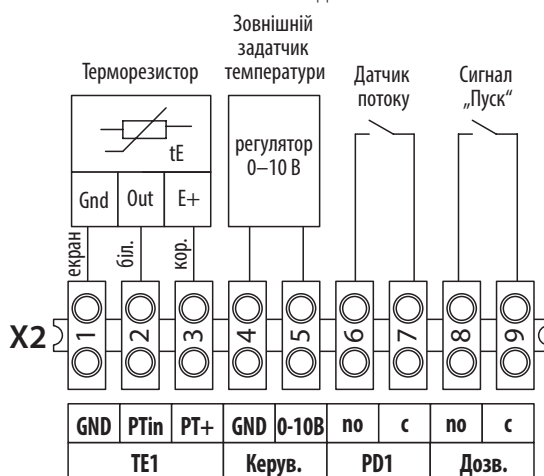
Схема зовнішніх підключень
