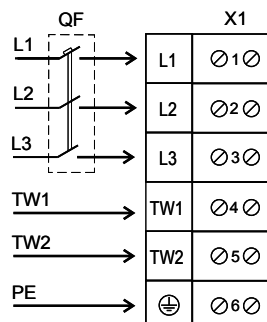
Схема підключення до електромережі OB, OBK, ВКФ з трифазним двигуном
