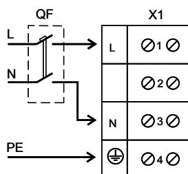
Схема підключення до електромережі OB, OBK, ВКФ, ОВП з однофазним двигуном
